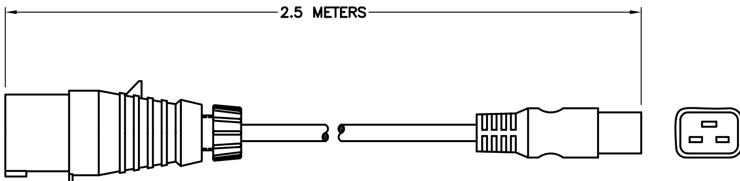
IEC 60320. C-19
