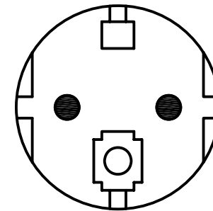
CEE 7-7 (SCHUKO)
