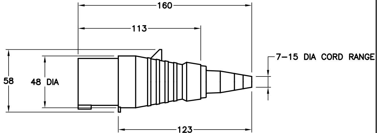
IEC 60309. 4H
