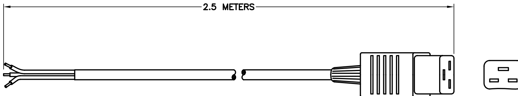
IEC 60320. C-19
